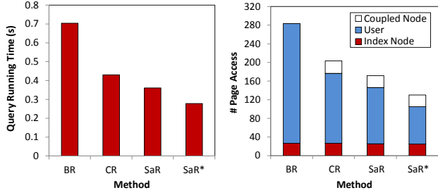
(c) GSGQ_{rkNN} ( k=100, c=4 ) (d) GSGQ_{rkNN} ( k=100, c=4 )
