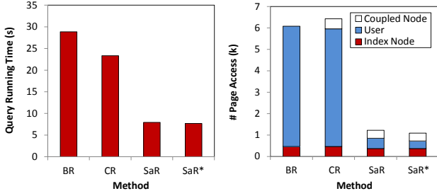
(c) GSGQ_{rkNN} ( k=20, c=2 ) (d) GSGQ_{rkNN} ( k=20, c=2 )
