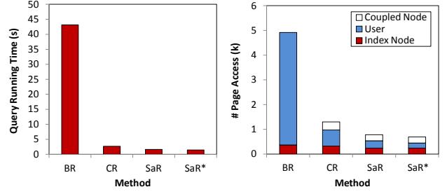
(c) GSGQ_{rkNN} ( k=100, c=4 ) (d) GSGQ_{rkNN} ( k=100, c=4 )
